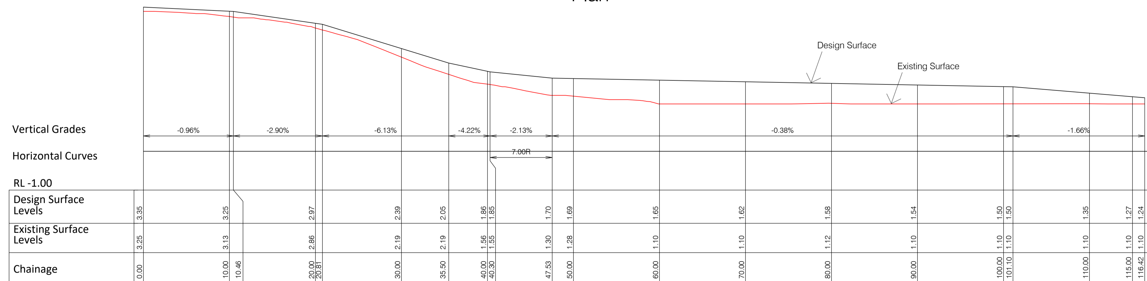
Longitudinal Section
